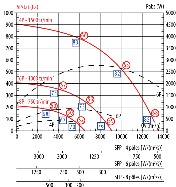
TEDH F400 560 TEDV F400 560
