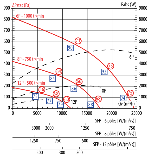
TEDH F400 810 TEDV F400 810
