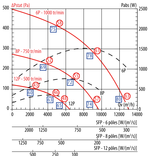
TEDH F400 630 TEDV F400 630
