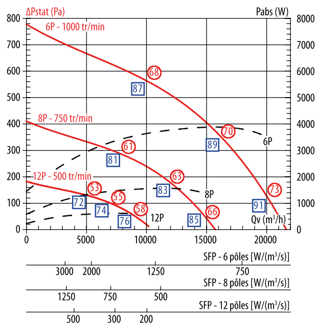
TEDH F400 760 TEDV F400 760
