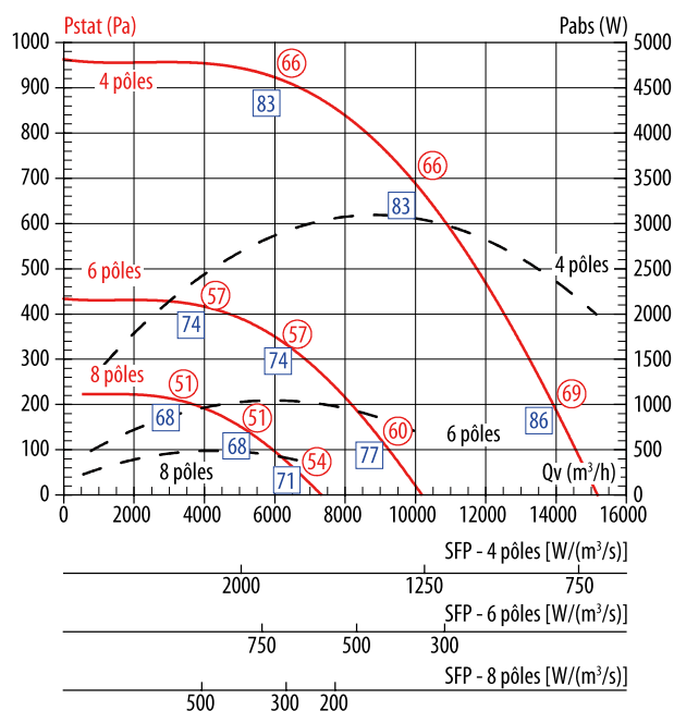
TEDH F400 600 TEDV F400 600
